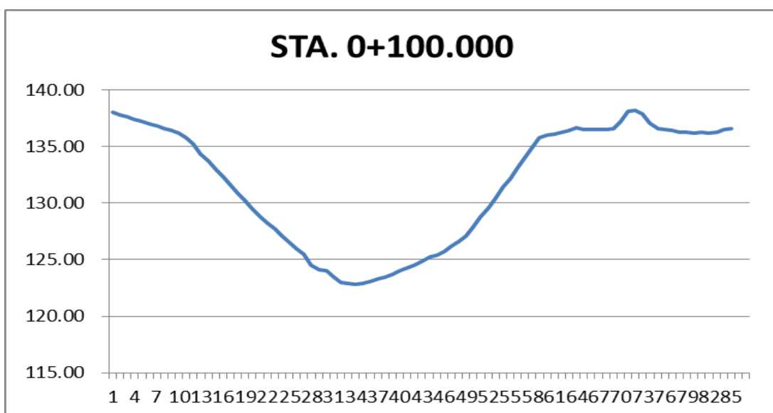
รูปที่ ข.6 หน้าตัดลำน้ำชี อบต.แสนชาติ (STA. 0+100.000)
