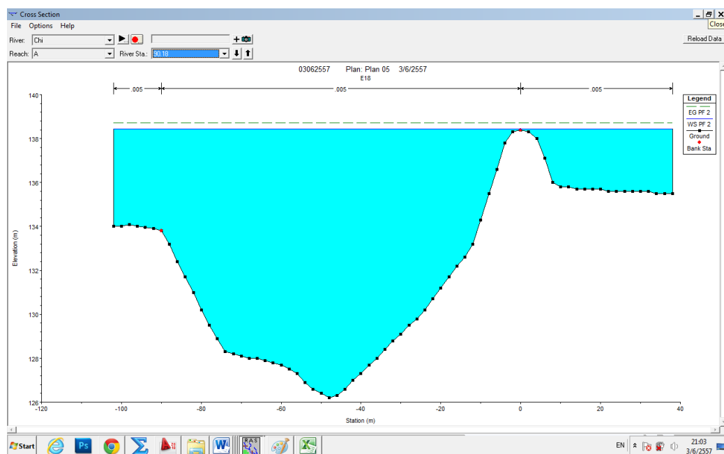
รูปที่ ง.2 หน้าตัดลำน้ำชี เทศบาลตำบลคงสิงห์ (STA. 0+057.601) ( T=50 , Q=1,800 )
