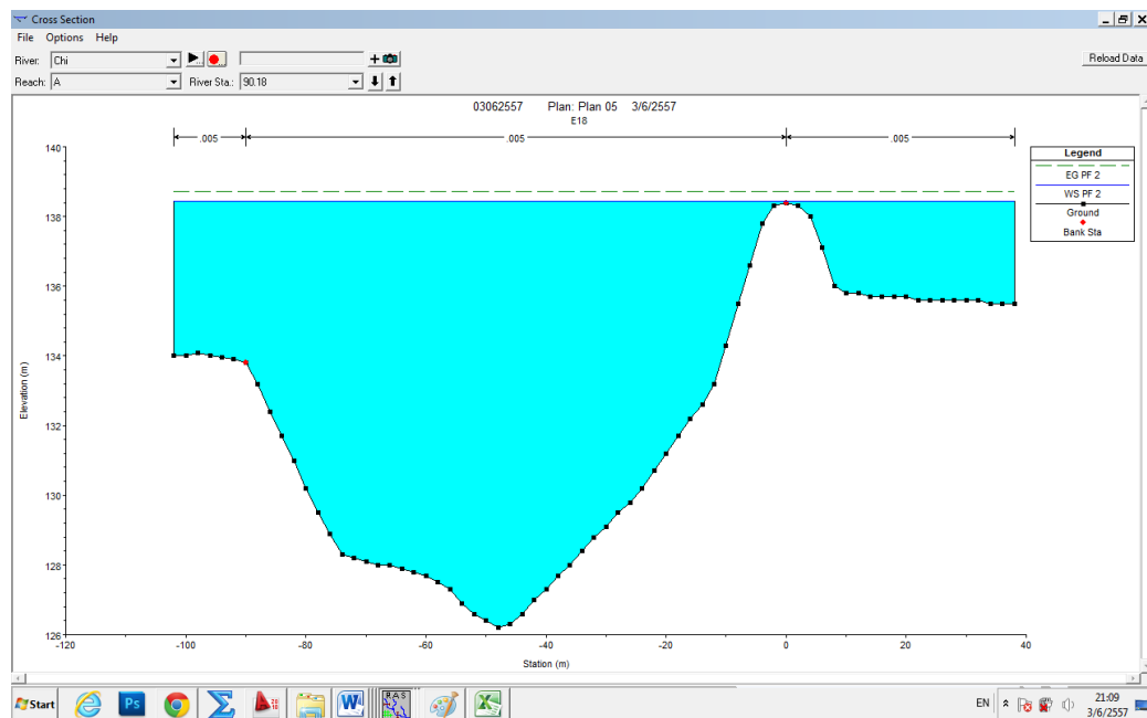
รูปที่ ก.3 หน้าตัดลำน้ำชี เทศบาลตำบลคงสิงห์ (STA. 0+100.000) (T=100 , Q=2,000)
