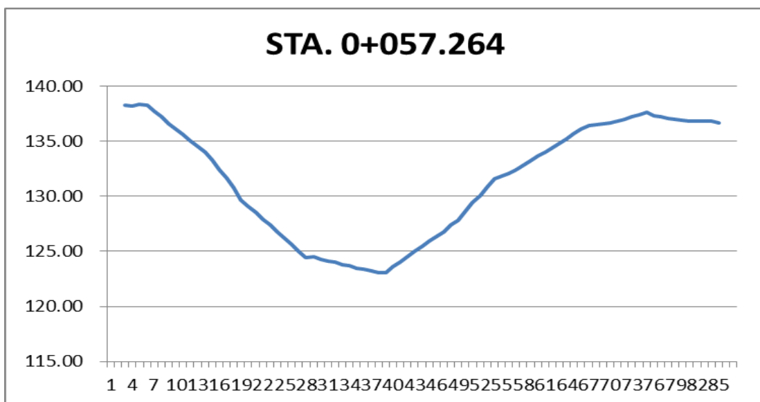
รูปที่ ข.5 หน้าตัดลำน้ำชี อบต.แสนชาติ (STA. 0+057.264)
